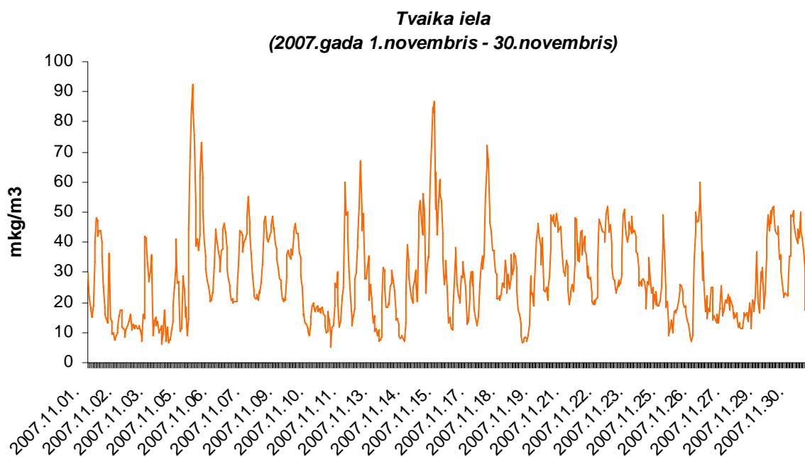
2.attēls. NO 2 stundas koncentrācijas stacijā Tvaika iela.
