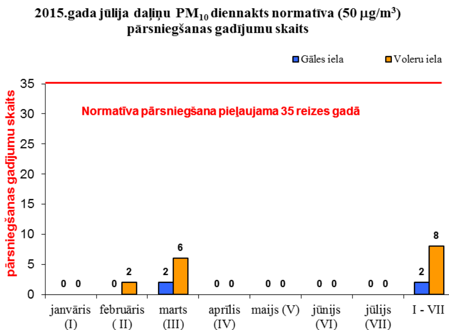
3.attēls. Daļiņu PM 10 diennakts normatīva pārsniegšanas gadījumi.
