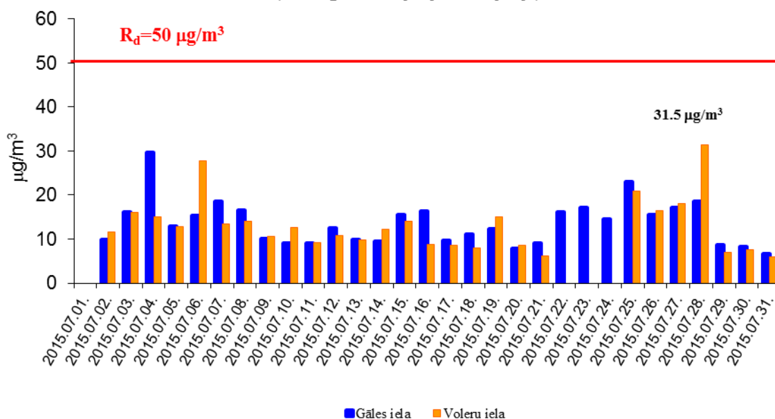
2.attēls. Daļiņu PM 10 diennakts koncentrācijas novērojumu stacijās Rīgas Brīvostas teritorijā.
