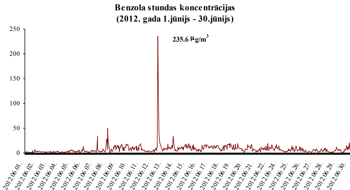
7.attēls. Benzola stundas koncentrācijas stacijā „Tvaika iela”.
