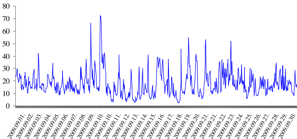
Slāpekļa dioksīda stundas koncentrācijas (2009. gada 1.septembris - 30. septembris)
