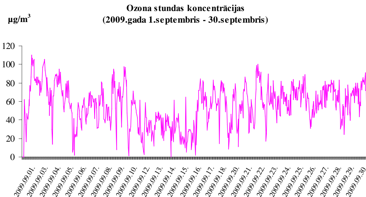
6. attēls. Ozona stundas koncentrācijas ( \mu\text{g}/\text{m}^3 ) stacijā BLB .
