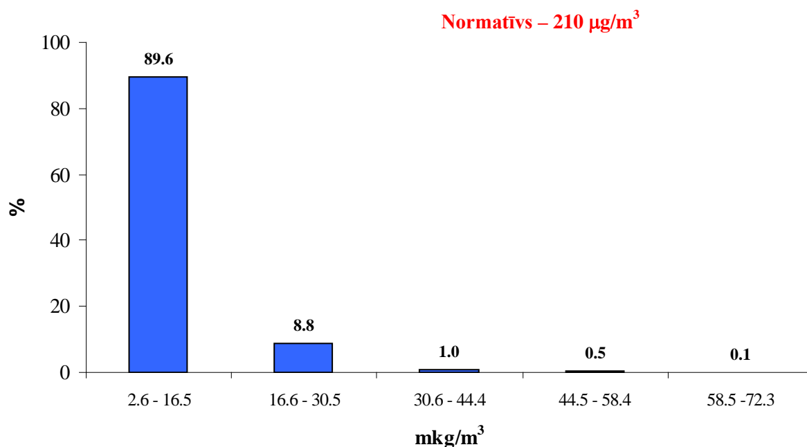
3. attēls. \text{NO}_2 stundas koncentrāciju ( \mu\text{g}/\text{m}^3 ) sadalījums stacijā BLB.
