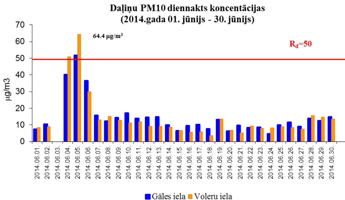
2.attēls. Daļiņu PM 10 diennakts koncentrācijas novērojumu stacijās Rīgas Brīvostas teritorijā.
