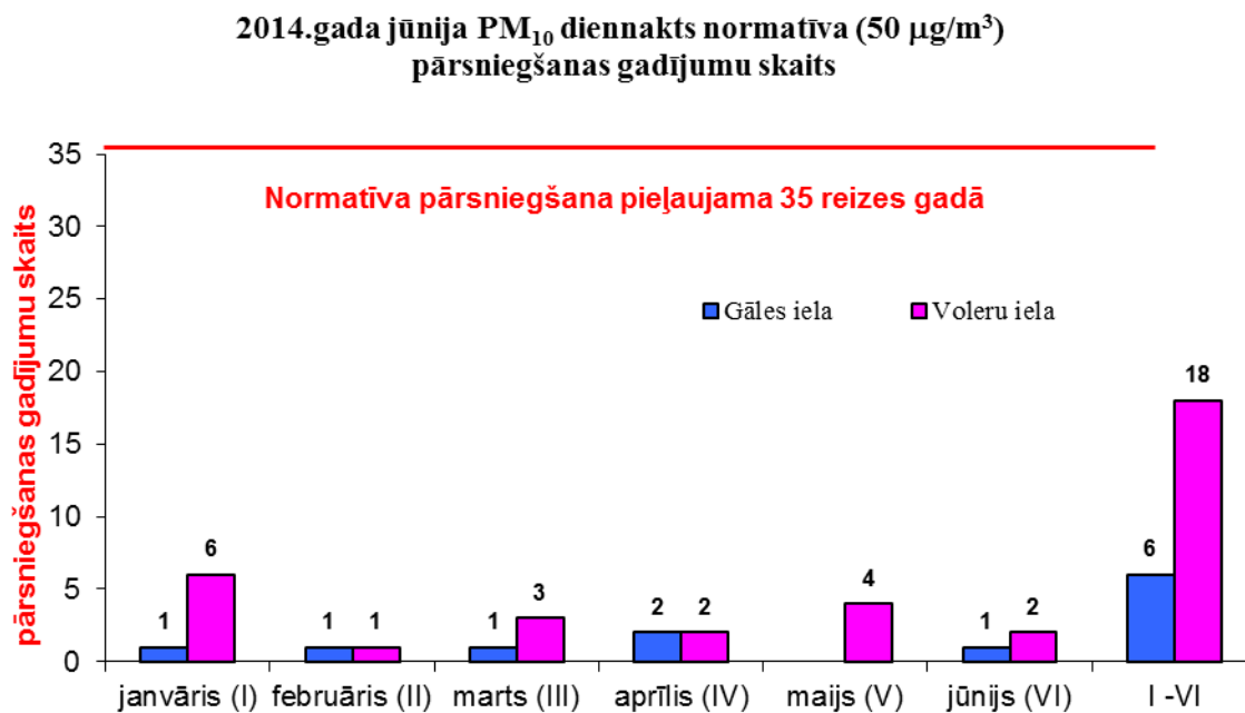
3.attēls. Daļiņu PM 10 diennakts normatīva pārsniegšanas gadījumi.
