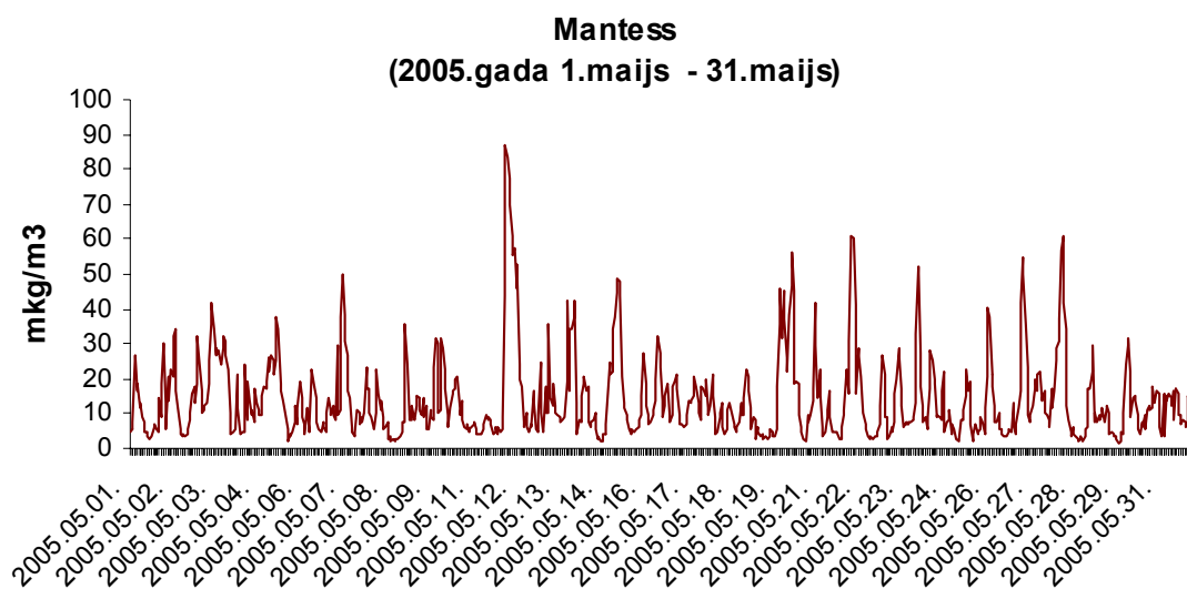
2.attēls. NO 2 stundas koncentrācijas stacijā Mantess.
