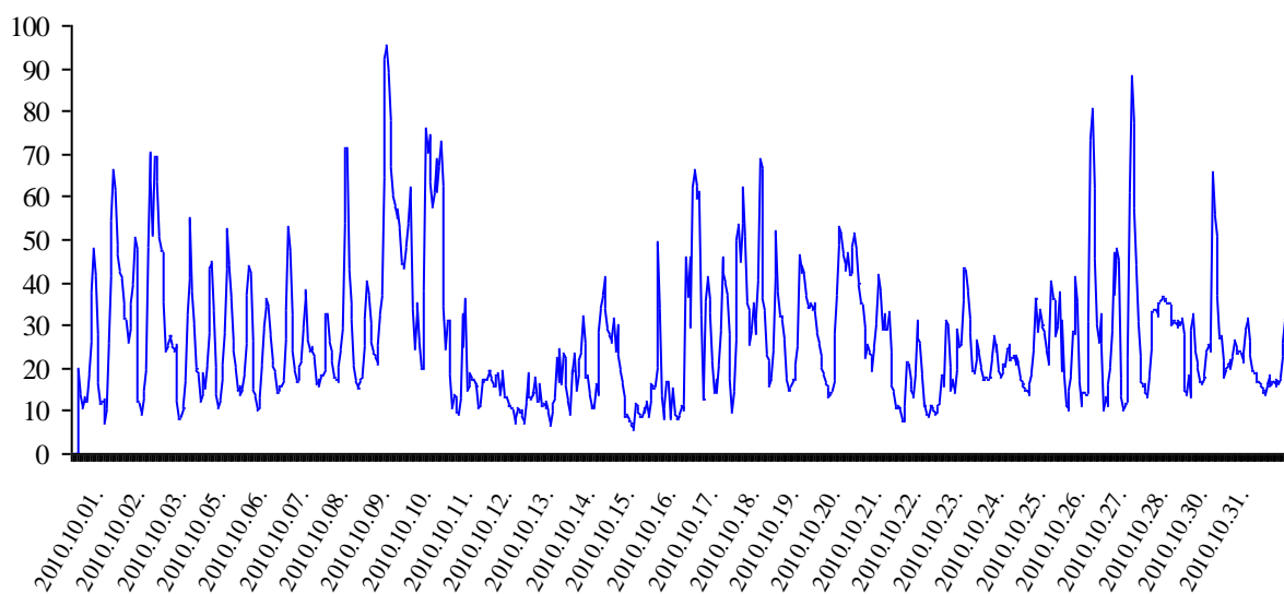
Slāpekļa dioksīda stundas koncentrācijas (2010. gada 1.oktobris - 31. oktobris)
