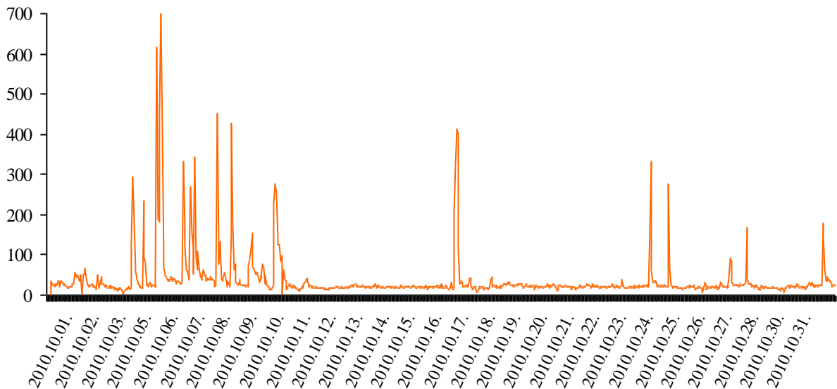
8.attēls. Toluola stundas koncentrācijas stacijā Man-Tess.
