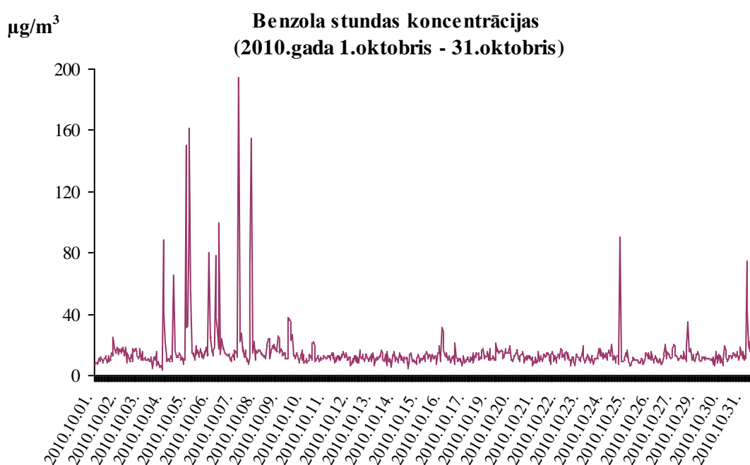
7.attēls. Benzola stundas koncentrācijas stacijā Man-Tess.
