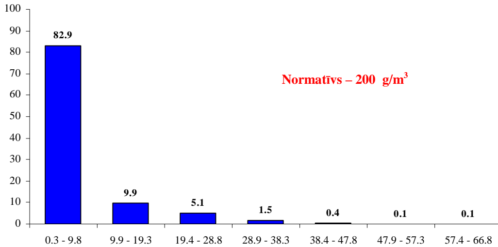
3. attēls. NO_2 stundas koncentrāciju ( g/m^3 ) sadalījums stacijā BLB.
