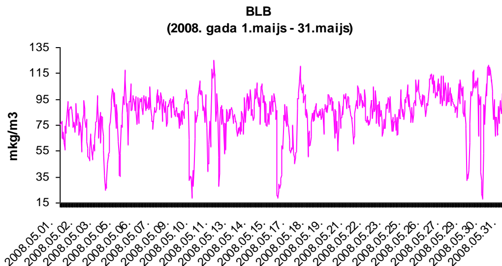
6. attēls. Ozona stundas koncentrācijas ( \mu\text{g}/\text{m}^3 ) stacijā BLB.
