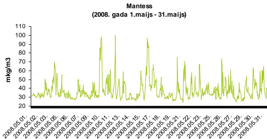
2.attēls. NO 2 stundas koncentrācijas stacijā Mantess.
