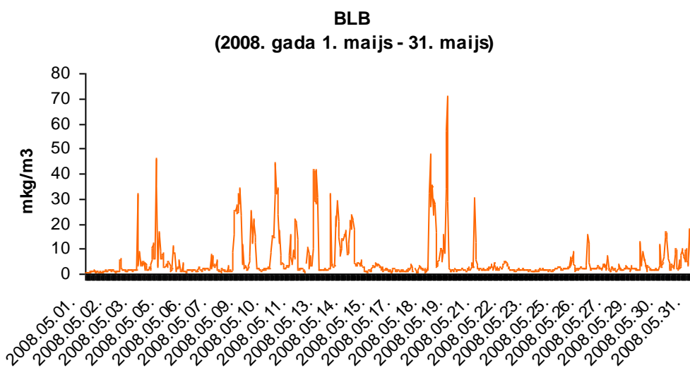
4.attēls.SO 2 stundas koncentrācijas stacijā BLB.
