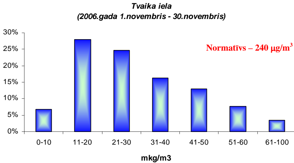
3. attēls. NO 2 stundas koncentrāciju (µg/m 3 ) sadalījums stacijā Tvaika ielā.
