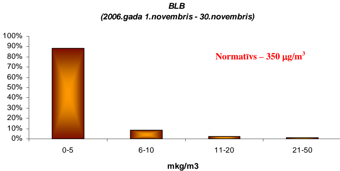
5. attēls. \text{SO}_2 stundas koncentrāciju ( \mu\text{g}/\text{m}^3 ) sadalījums stacijā Mīlgrāvis.
