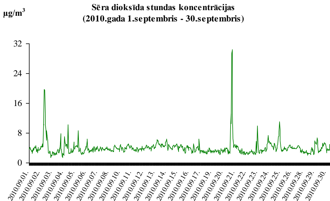
4.attēls. \text{SO}_2 stundas koncentrācijas stacijā Man-Tess.
