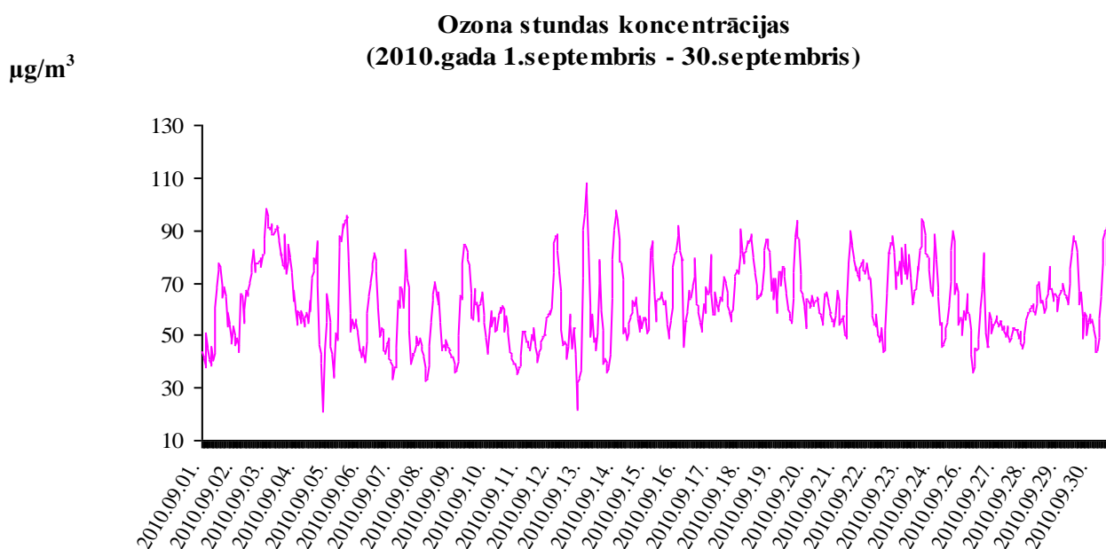
6. attēls. Ozona stundas koncentrācijas ( \mu\text{g}/\text{m}^3 ) stacijā Man-Tess.
