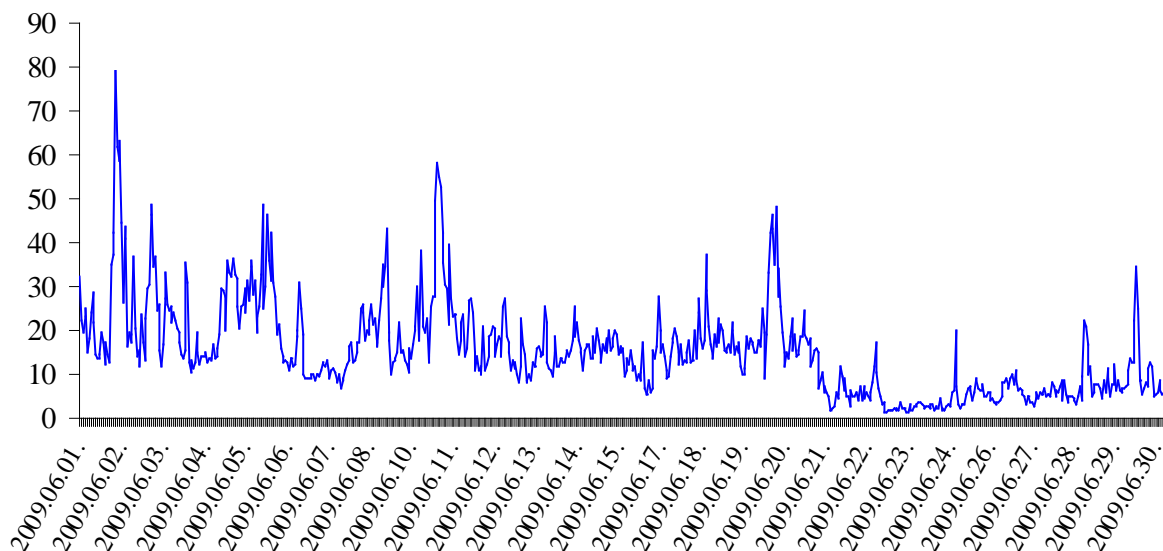
Slāpekļa dioksīda stundas koncentrācijas (2009. gada 1.jūnijs - 30. jūnijs)
